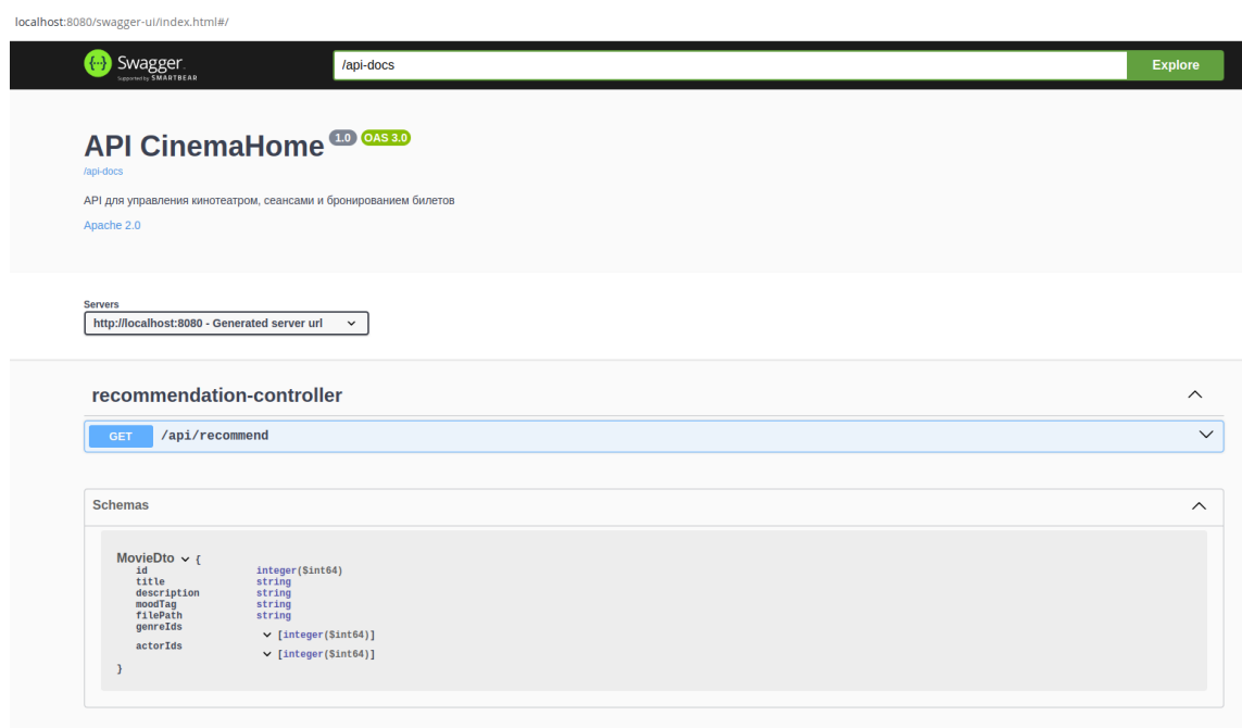
Рисунок 12 — Swagger UI
